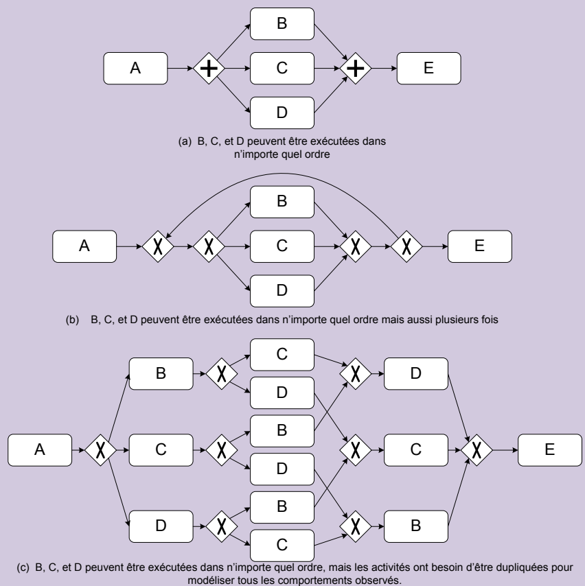
Figure 6: Un exemple illustrant des problèmes quand la concurrence (c'est-à-dire AND-splits/joins) ne peut pas être exprimée directement. Dans l'exemple seulement trois activités (B, C et D) sont en concurrence. Imaginez les modèles de procédé résultant quand il y a 10 activités en concurrence ( 2^{10} = 1024 états et 10! = 3,628,800 séquences d'exécution possibles).
